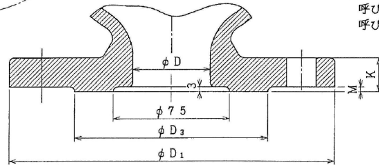
呼び径 ※φ50のフランジ形状
