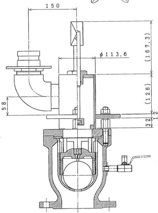
玉押し器取付参考図
