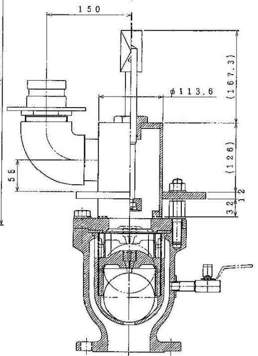
玉押し器取付参考図
