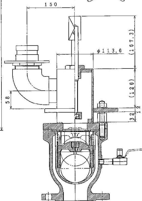
玉押し器取付参考図
