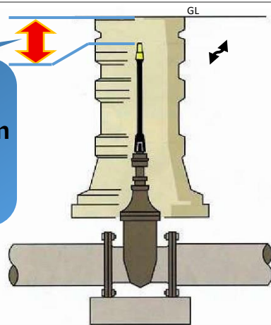
図 1 継足しキー装着例
