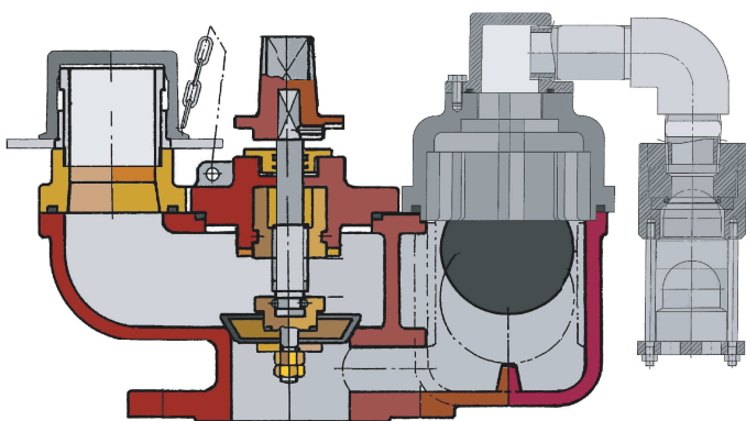
WMC 型 汚水流入防止機能付 空気弁付消火栓 定価 ¥178,000-
