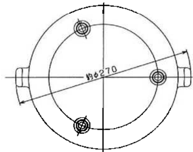
空気弁上面
