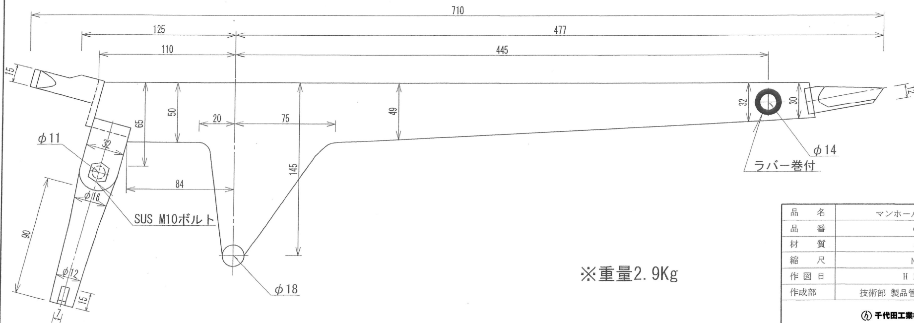
側面図
