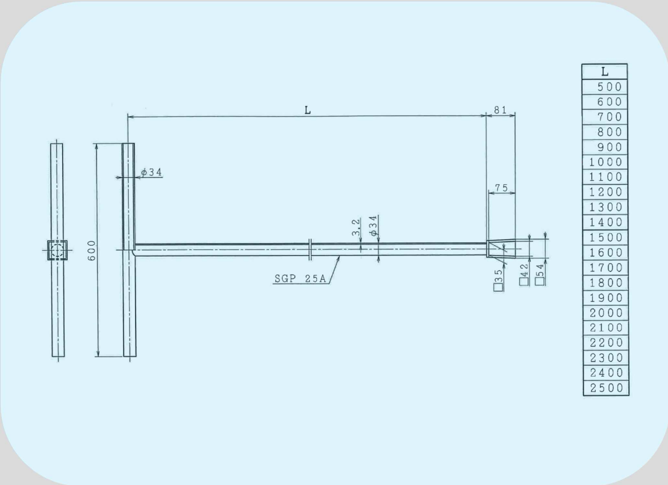
CHT外形図
