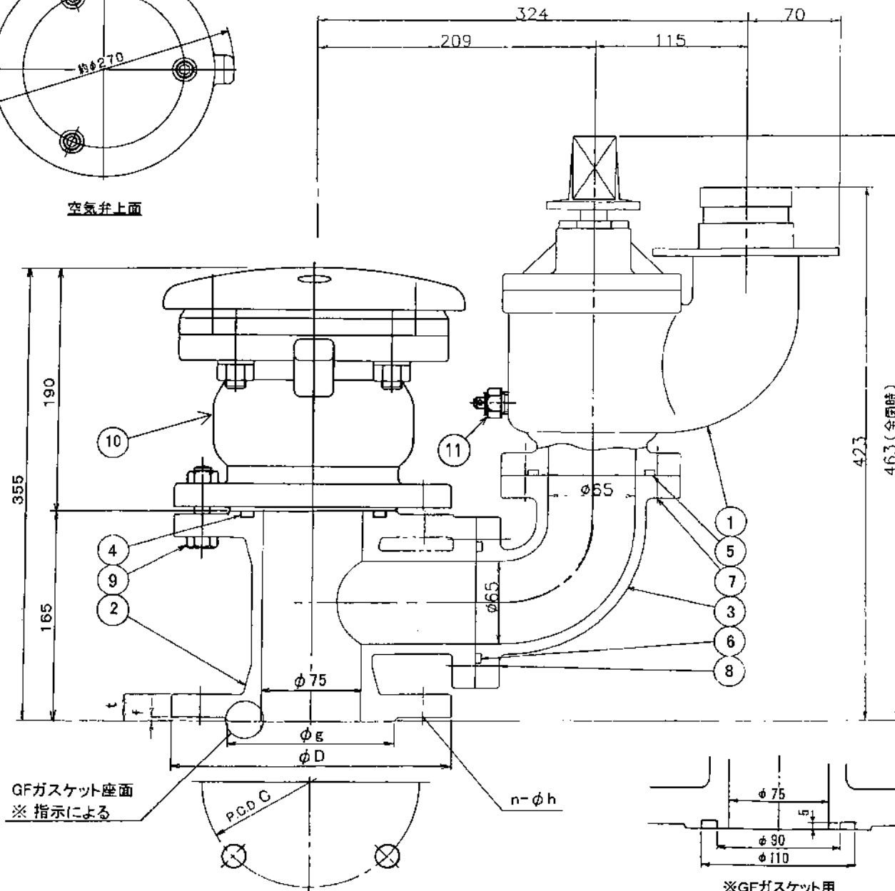
※GFガスケット用 フランジ寸法図
