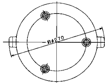
空気弁上面
