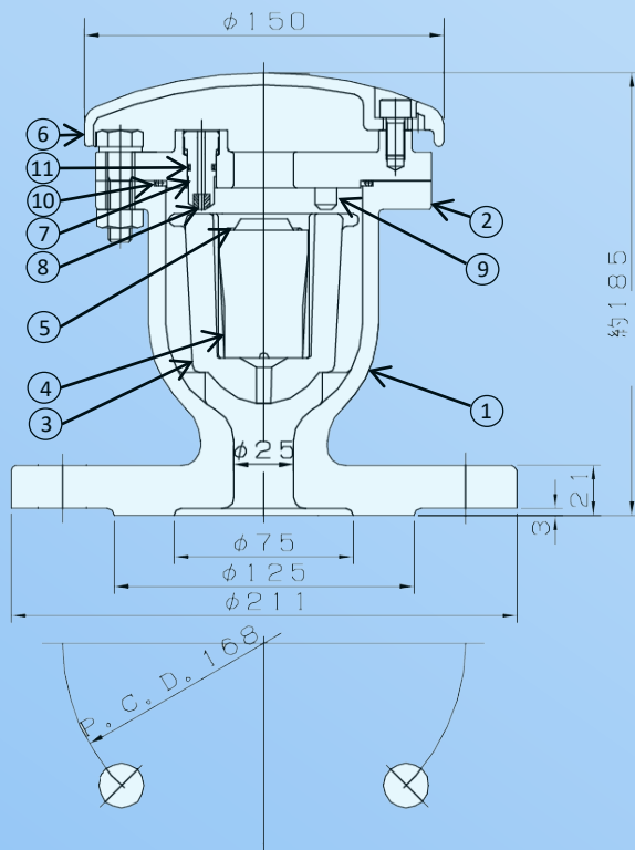
外径寸法
