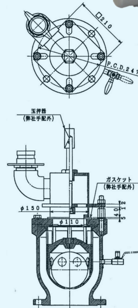
玉押器取付参考図
