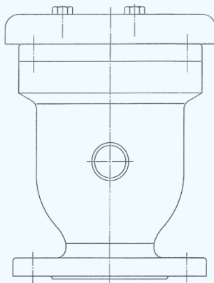
外径寸法
