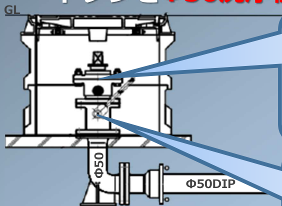
\Phi 50 洗浄栓
