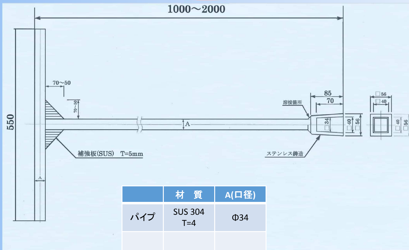
外形図
