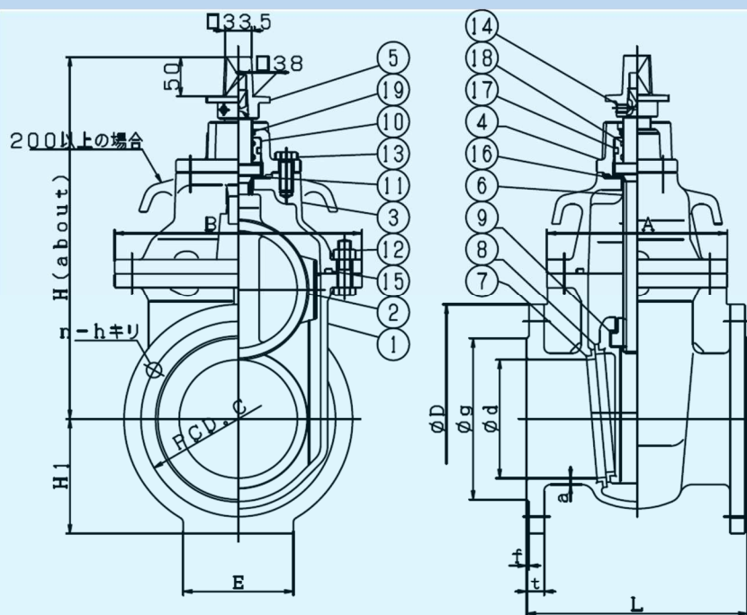
外形図 φ50～φ300
