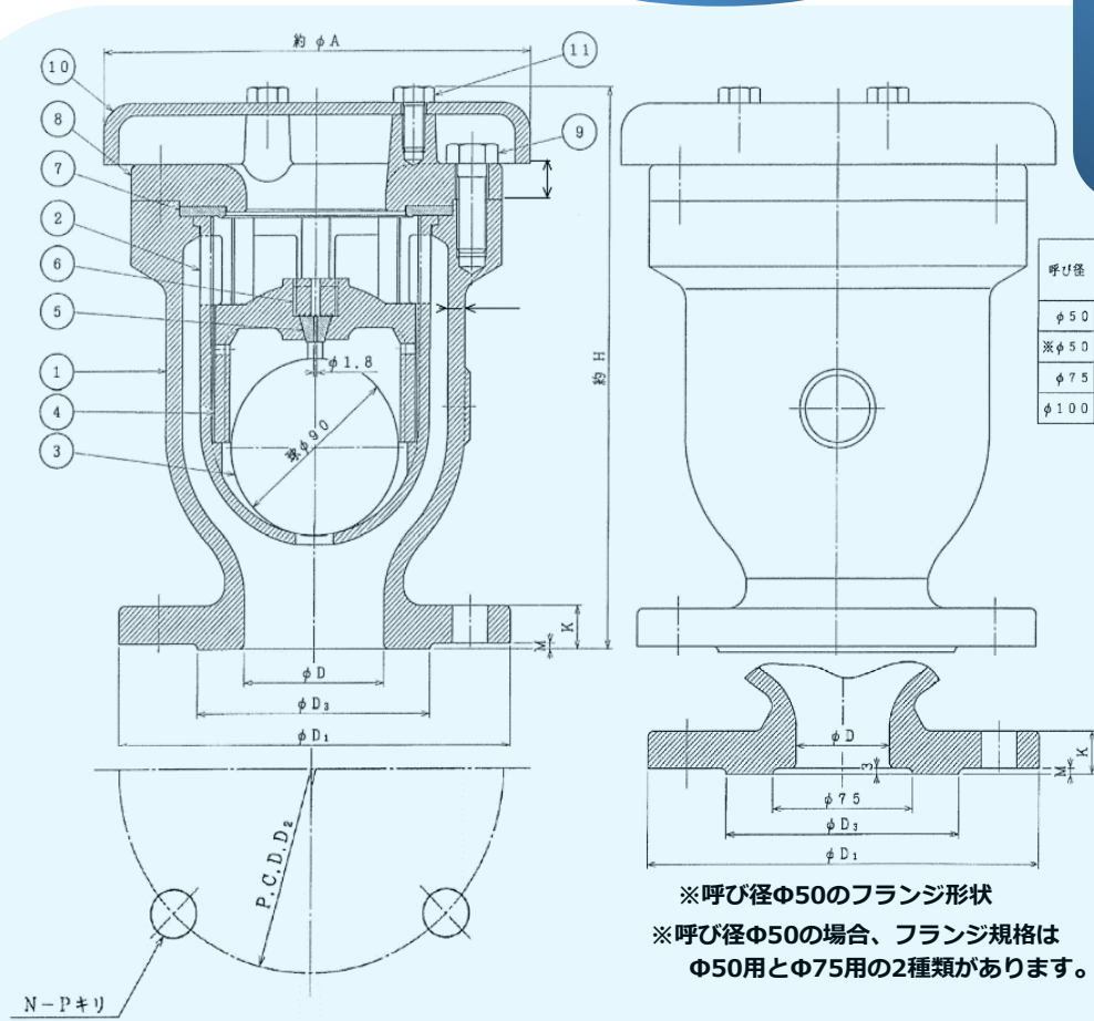
外径寸法例
