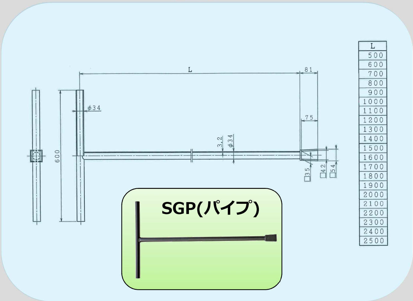
CHT外形図
