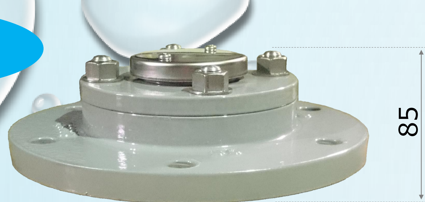
MC空気弁 Φ150xΦ25
