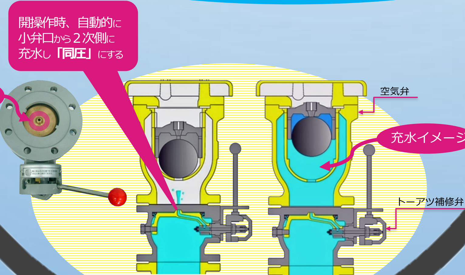
トーアツ補修弁の開閉 操作（充水）イメージ
