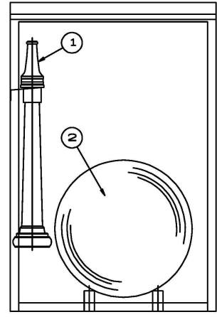
内部格納図
