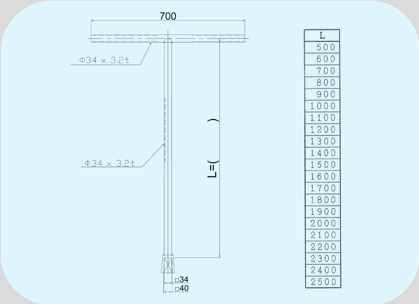
CHT外形図
