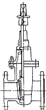
2 種・3 種（ロング形）
