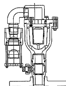
汚水流入防止型
