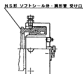
NS受口用カバー
