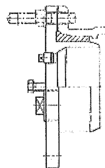
GX 受口用 カバー
