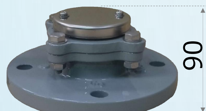
MC空気弁 Φ75×Φ25
