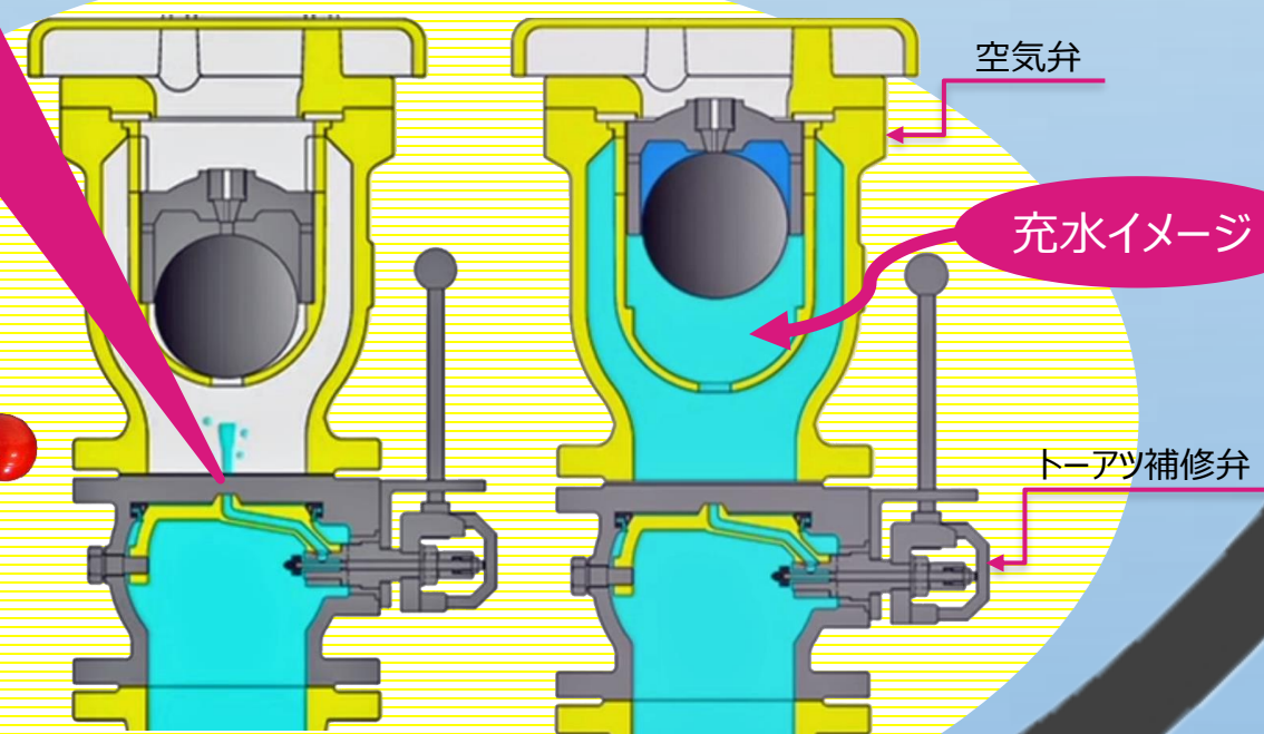
トアツ補修弁の開閉 操作（充水）イメージ
