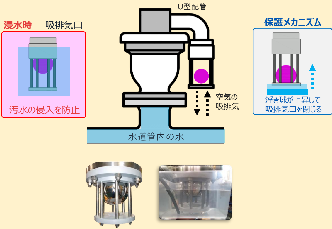
汚水流入防止ユニットの動作
