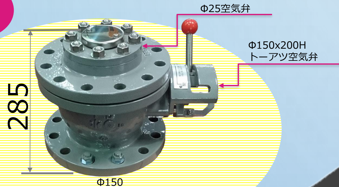
Φ25空気弁
