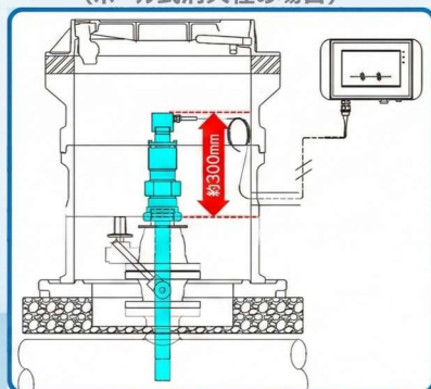
ULSONA流量計の設置イメージ図 (ボール式消火栓の場合)
