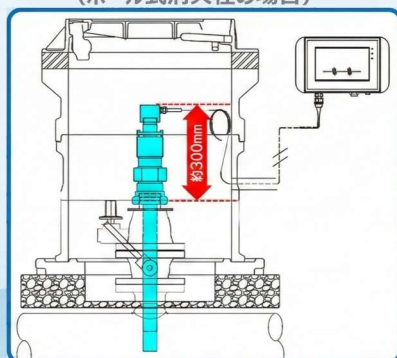
ULSONA流量计の設置イメージ図 (ボール式消火栓の場合)
